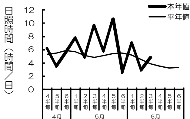
図 2 日照時間の推移（アメダス、佐倉）
