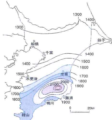
図4-3 年平均降水量 1979~1990年の平均(基準年値)。ただし、銚子は1986年以降観測点移動。(単位: mm)
