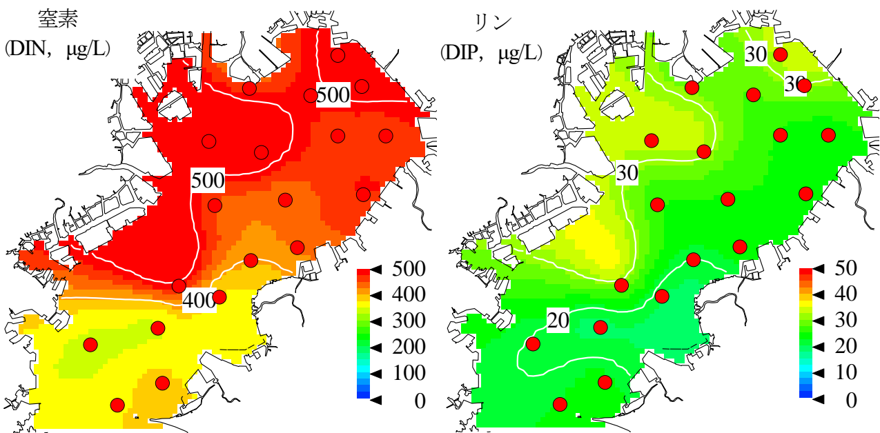
図3 表層の栄養塩濃度の分布
