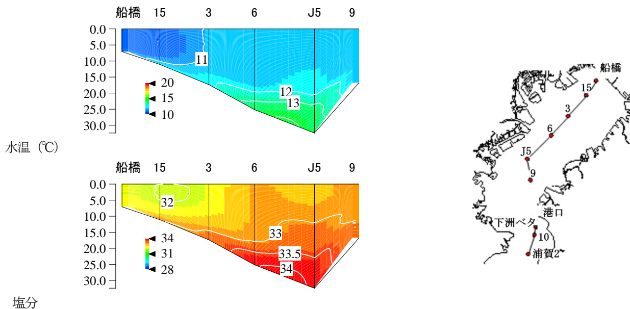
図2 縦断面の水温・塩分の鉛直分布 (上:水温, 下:塩分, 右:調査ライン)
