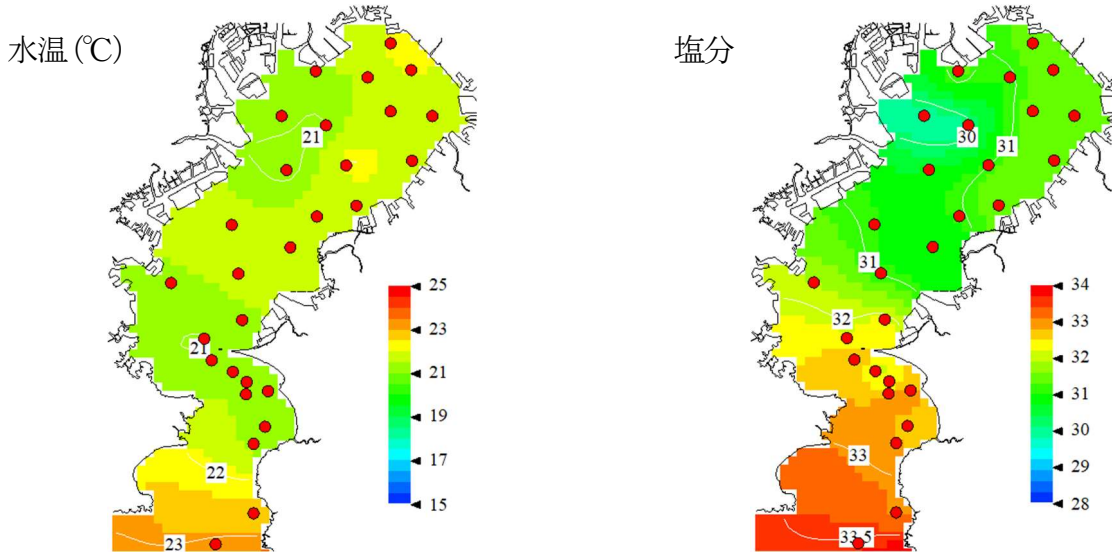
図1 表層の水温・塩分
