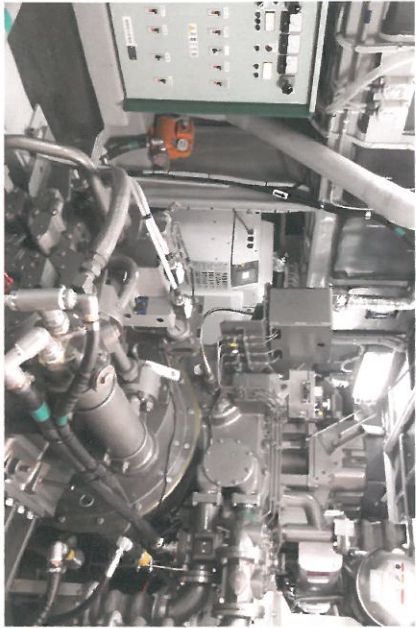
機関室
