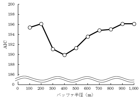
第3図 各森林占有率のバッファ半径におけるベストモデルの AIC
