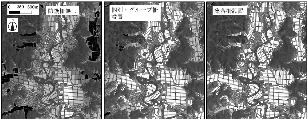
第4図 防護柵無し、個別・グループ柵、集落柵設置を仮定し作成したイノシシ水稻被害発生リスクマップ（一部）
