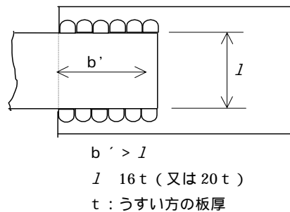
図 6-2-3 側面すみ肉溶接の重ね代( b' )
