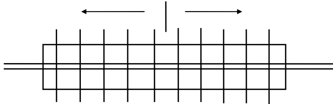
図5 - 4 - 1 ボルト締め付け順序
