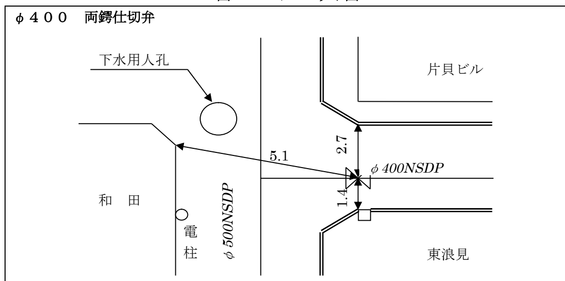
図-2 オフセット図
