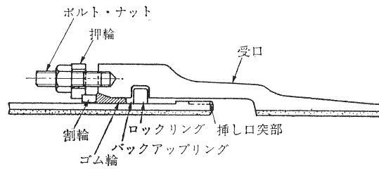
図 5.8 S形鋳鉄管の接合
