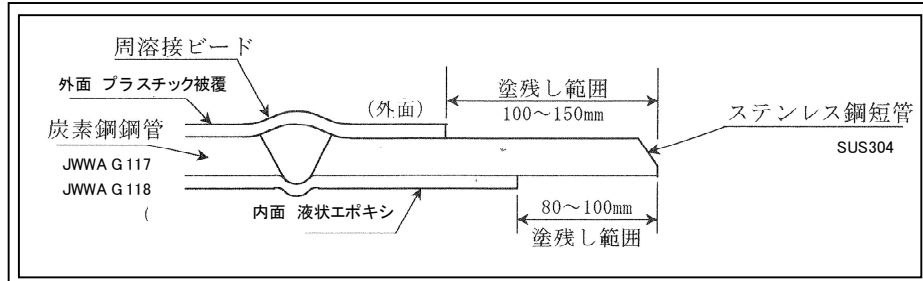
図 8.2 管端内外面塗覆装の仕上げ
