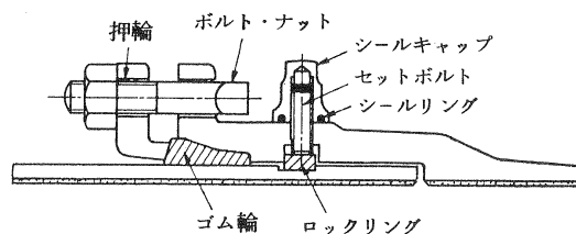
図 5.3 K F形鋳鉄管の接合
