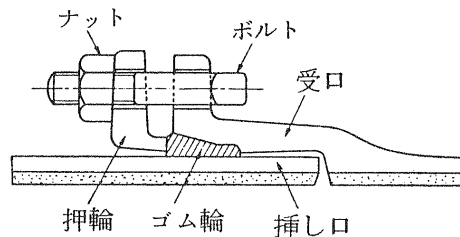
図 5.1 K形鋳鉄管の接合
