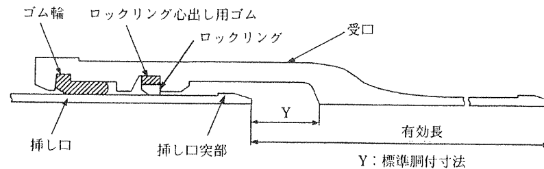
図 5.9 NS形鋳鉄管（直管）の接合
