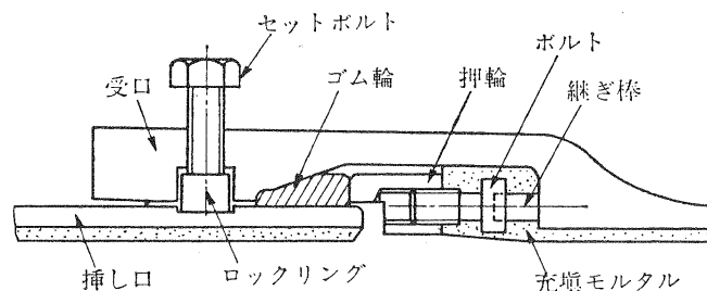
図 5.5 UF形铸铁管の接合
