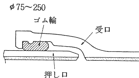
図 5.2 T形鋳鉄管の接合
