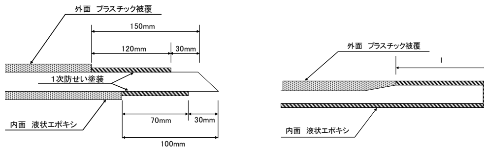
図 6.2 管端内外面塗覆装の仕上げ
