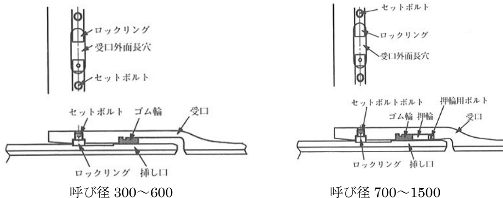
図 5.10 PN形鋳鉄管の接合
