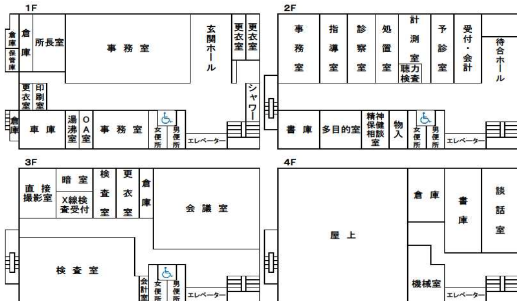
庁舎平面図
