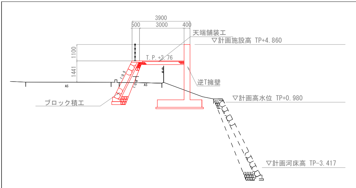
代表断面図
