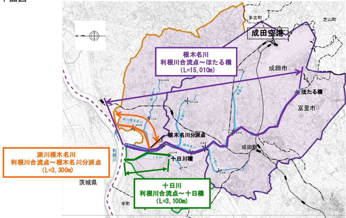
計画平面図
