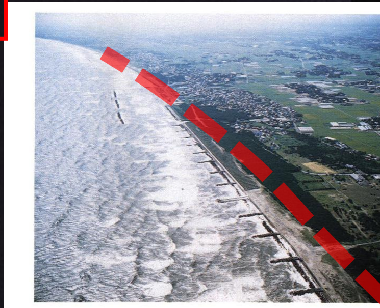
写真-5 北九十九里海岸の小突堤群と離岸堤および1, 2号ヘッドラン
