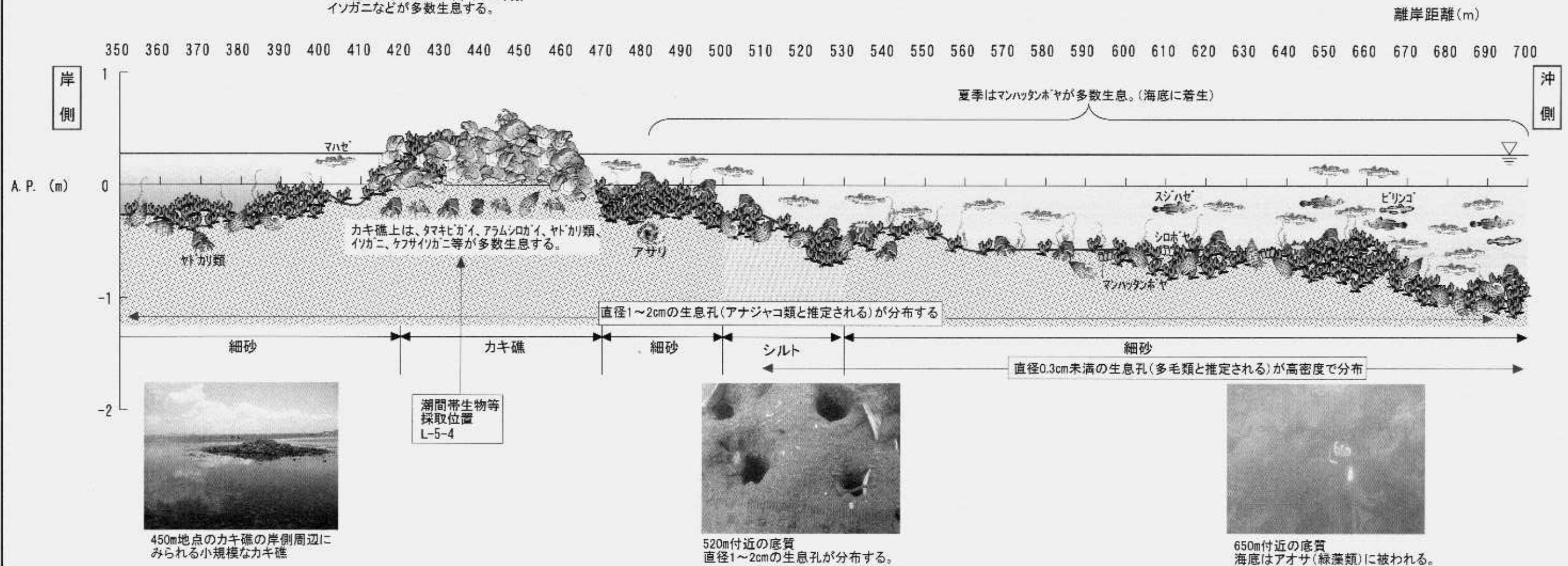
カキ礁を形成するマガキ 層状に積み重なっている。(450m付近)
