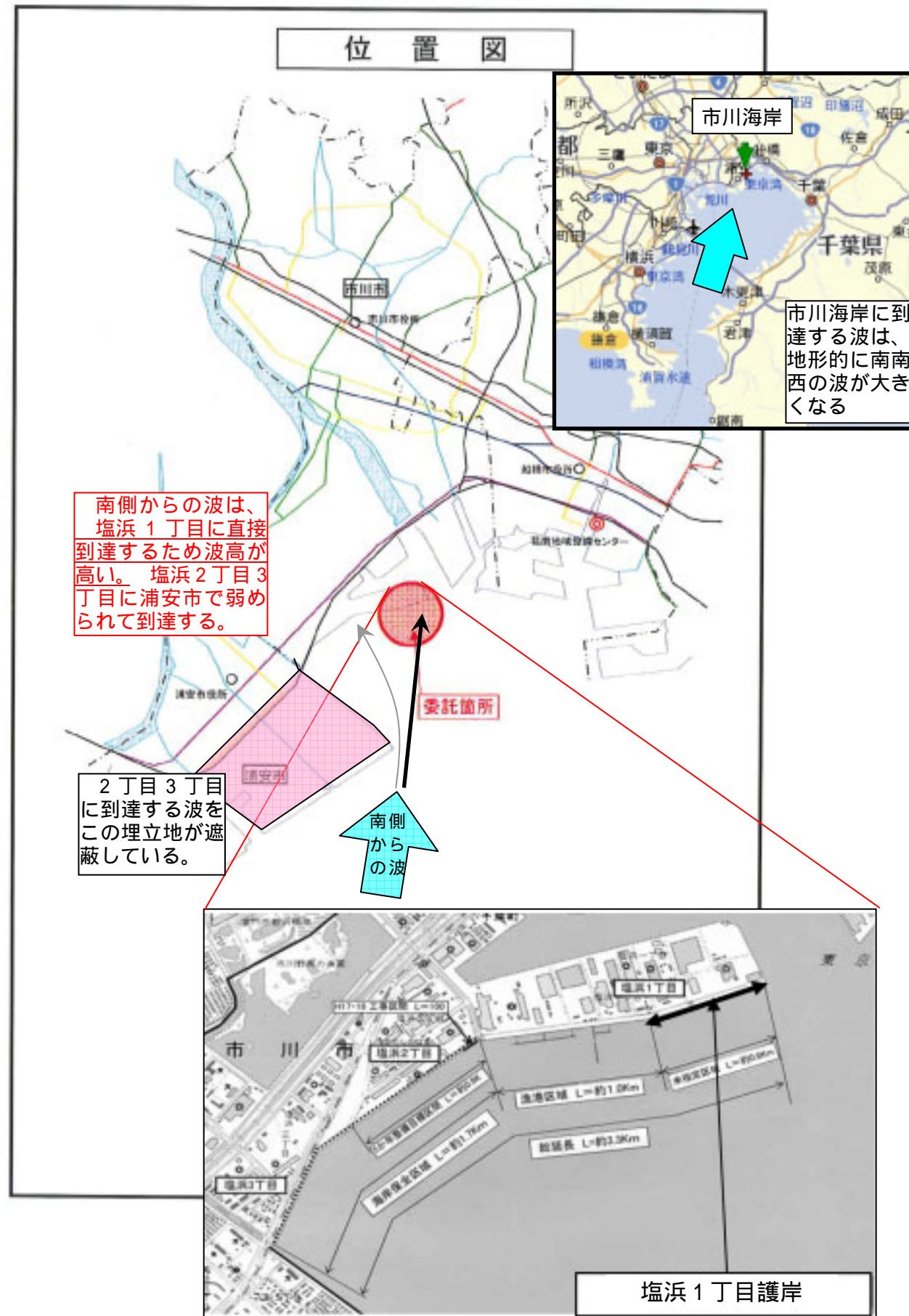
添付資料-2 塩浜1丁目に到達する波浪の特性
