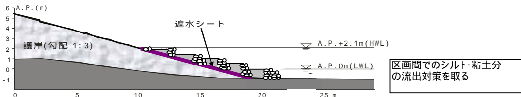
【断面】
