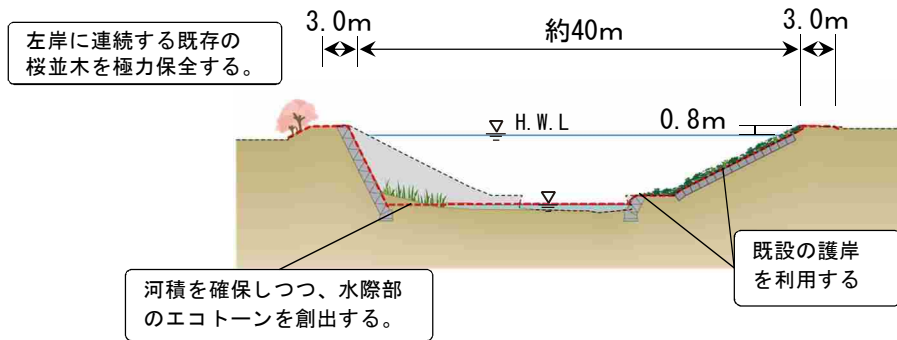
■ 河道改修代表断面（治水断面および環境に配慮した断面）イメージ
