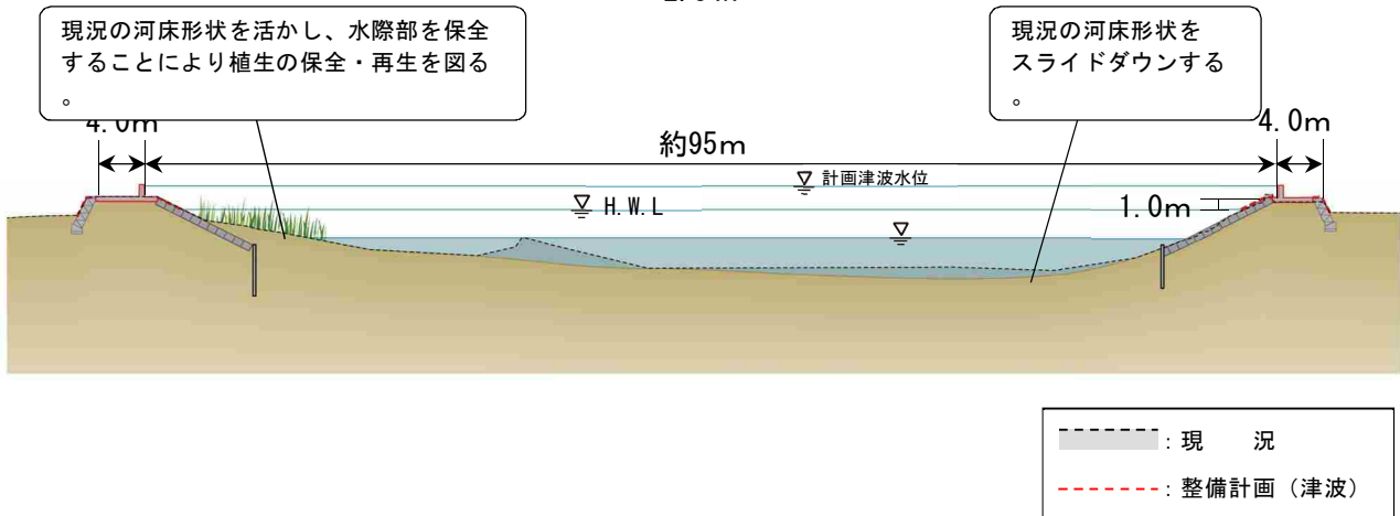
■ 河道改修代表断面（治水断面（津波対策含む）および環境に配慮した断面）イメージ
