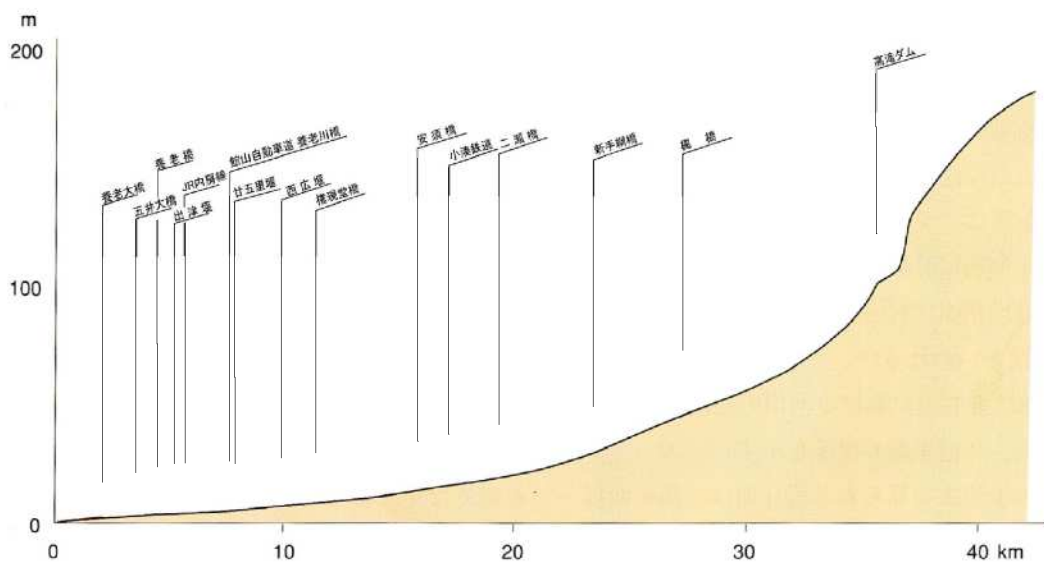
図 1-5 養老川の河床勾配
