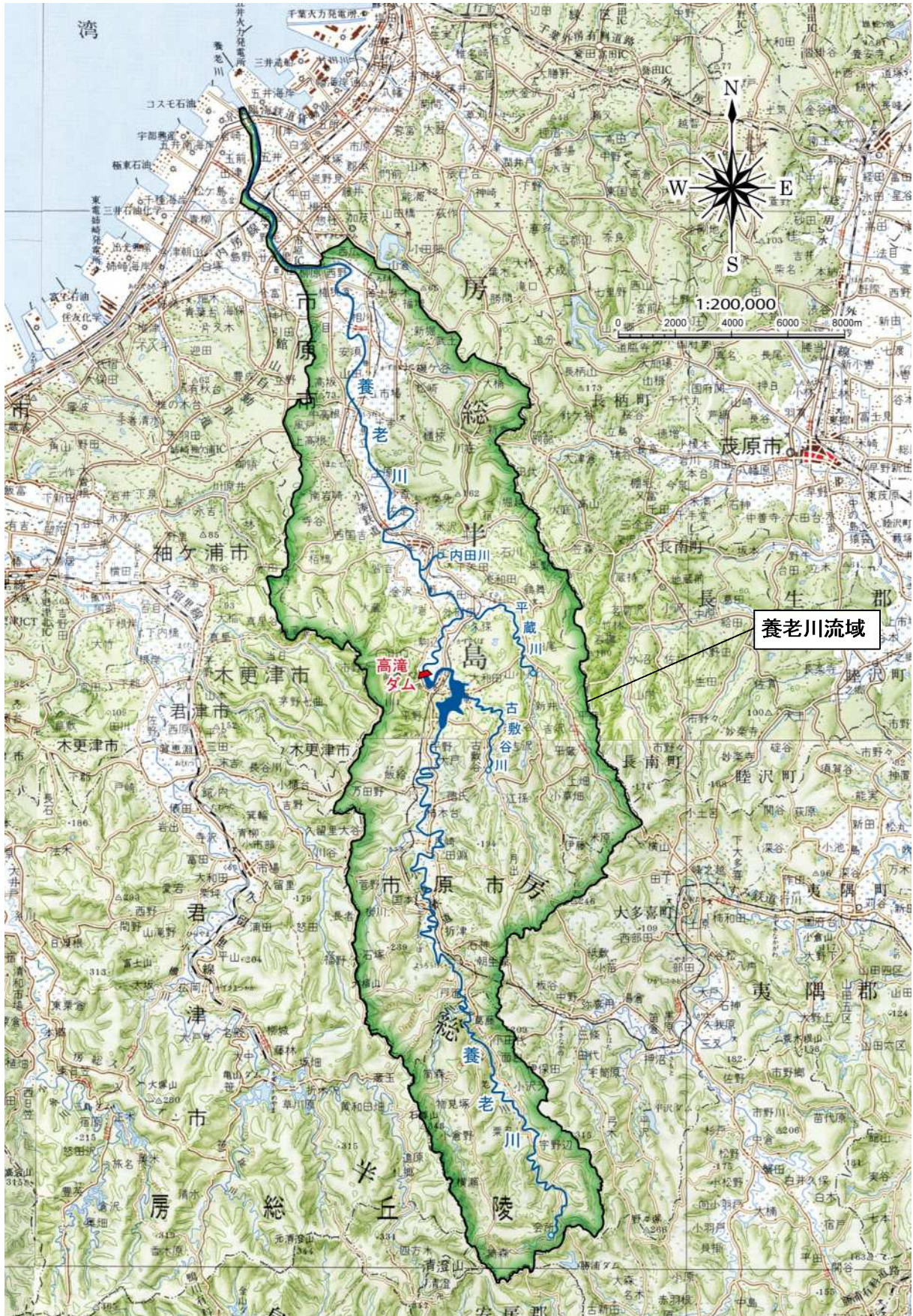
図 1-2 養老川流域図
