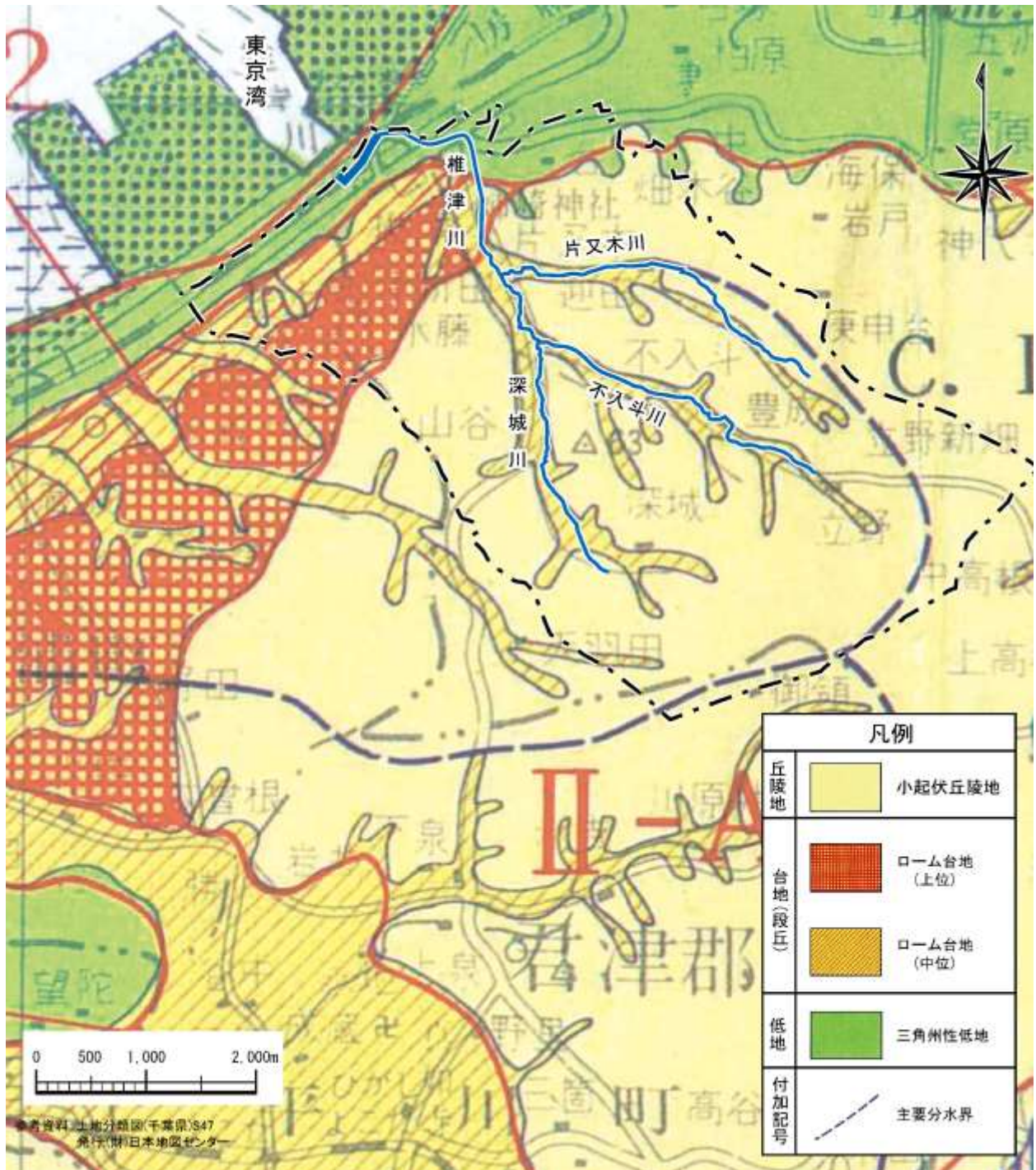
图 1.5 椎津川流域近傍の地質図
