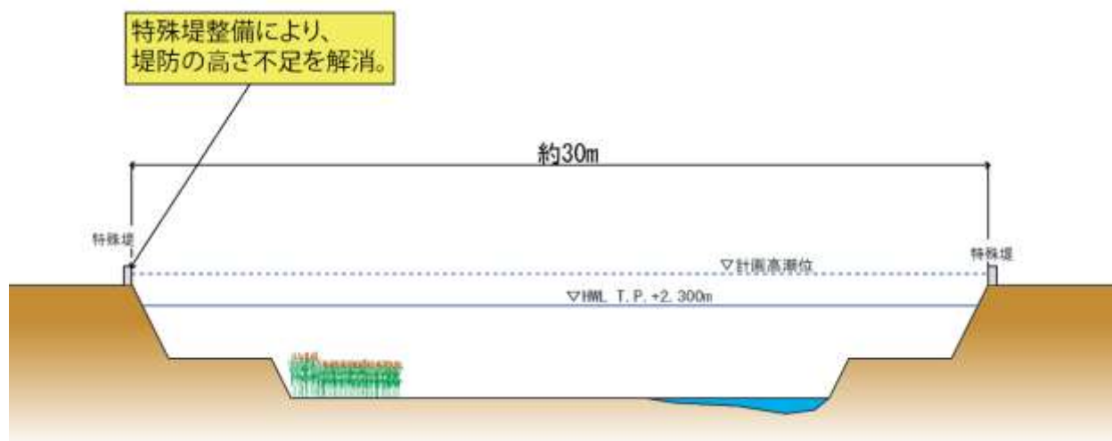
図 4.3 代表横断面図 JR内房線下流～横町橋区間 (No. 15 地点)
