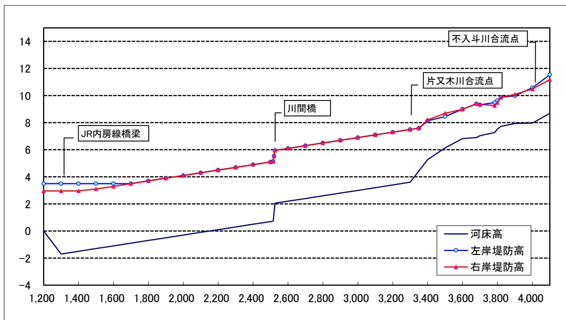
図 1.13 椎津川 現況河道 縦断模式図
