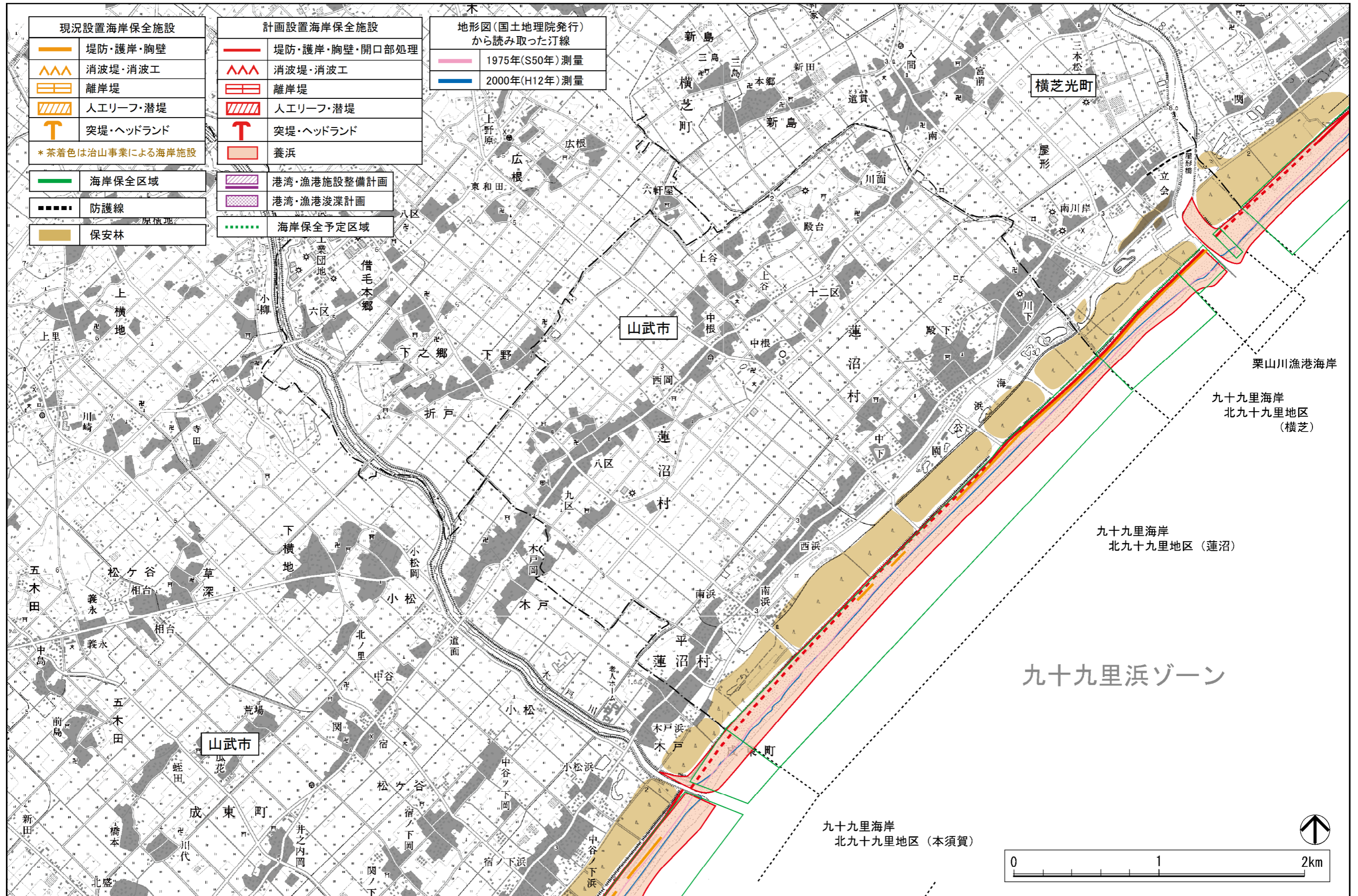
「この地図は、国土地理院長の承認を得て、同院発行の数値地図25000(地図画像)を複製したものである。(承認番号 平成15総複、第212号)」 図- 4-2(5) 施設整備計画(九十九里浜ゾーン)
