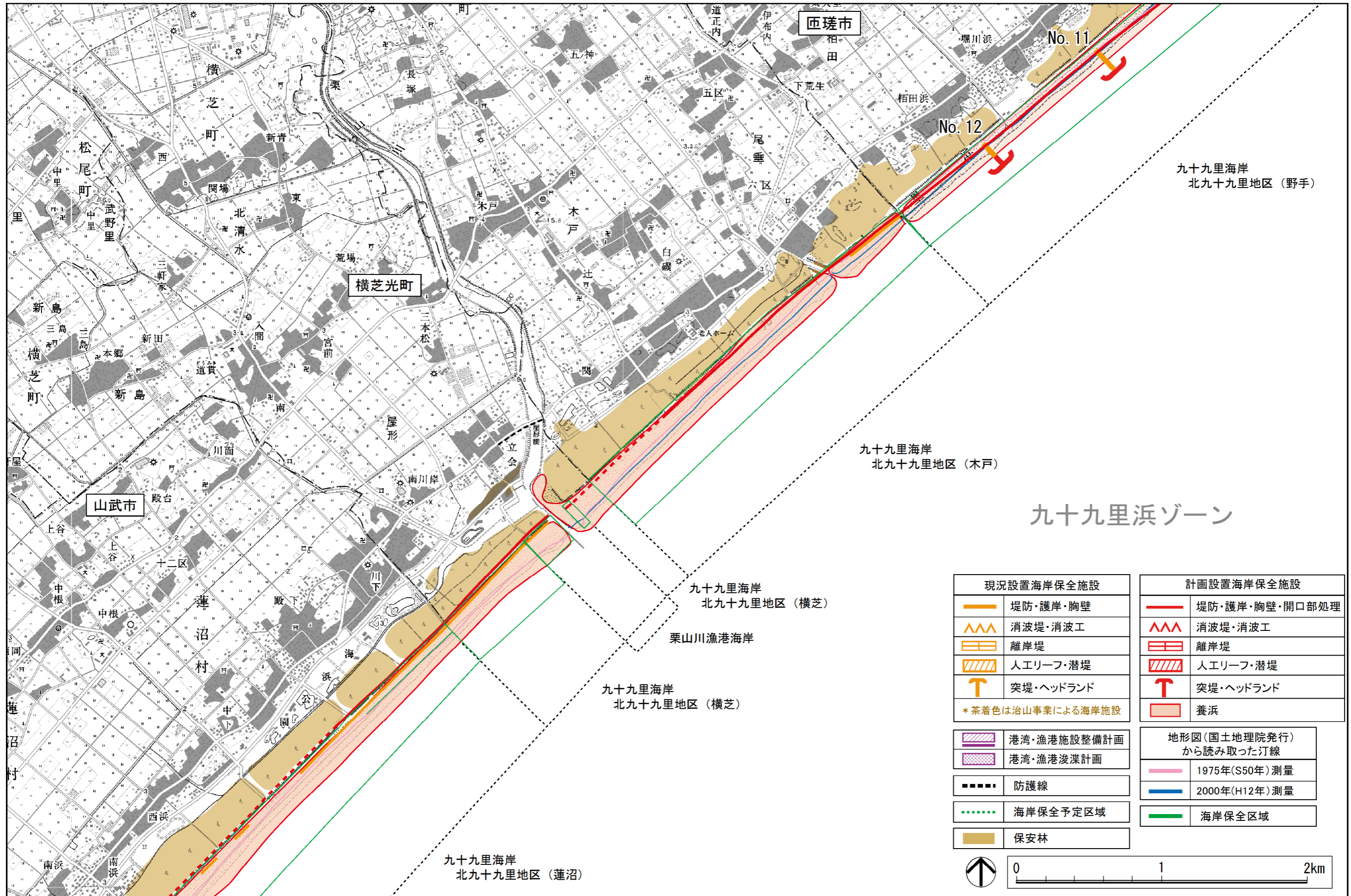
「この地図は、国土地理院長の承認を得て、同院発行の数値地図25000(地図画像)を複製したものである。(承認番号 平成15総複、第212号)」 図- 4-2(4) 施設整備計画(九十九里浜ゾーン)
