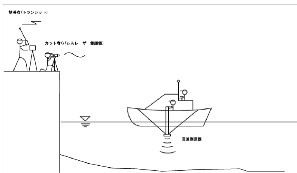
図 1.4.1 測量概要図
