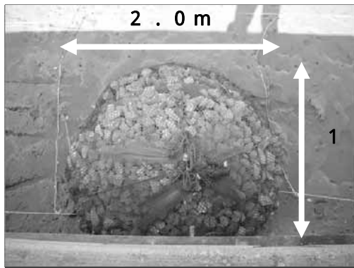
試験施工した袋詰め捨て石
