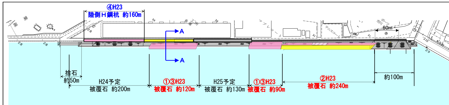
A-A断面
