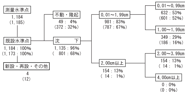
図 2-10-2 地盤変動量別・水準点数 ( ) 内は13年度
