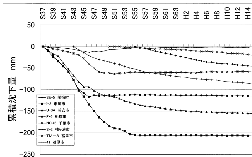
図2-10-1 主要地点の経年地盤変動
