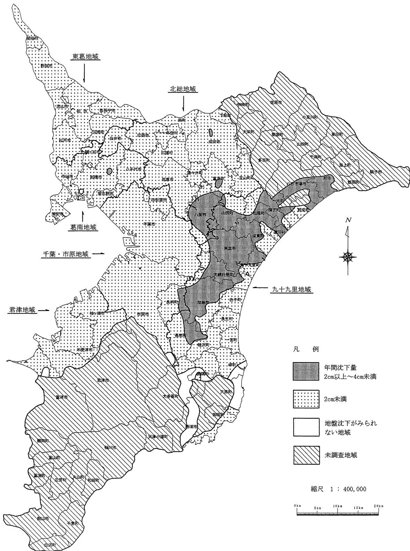
図2-10-3 千葉県水準基標変動図（1年間変動図）（14年1月～15年1月）
