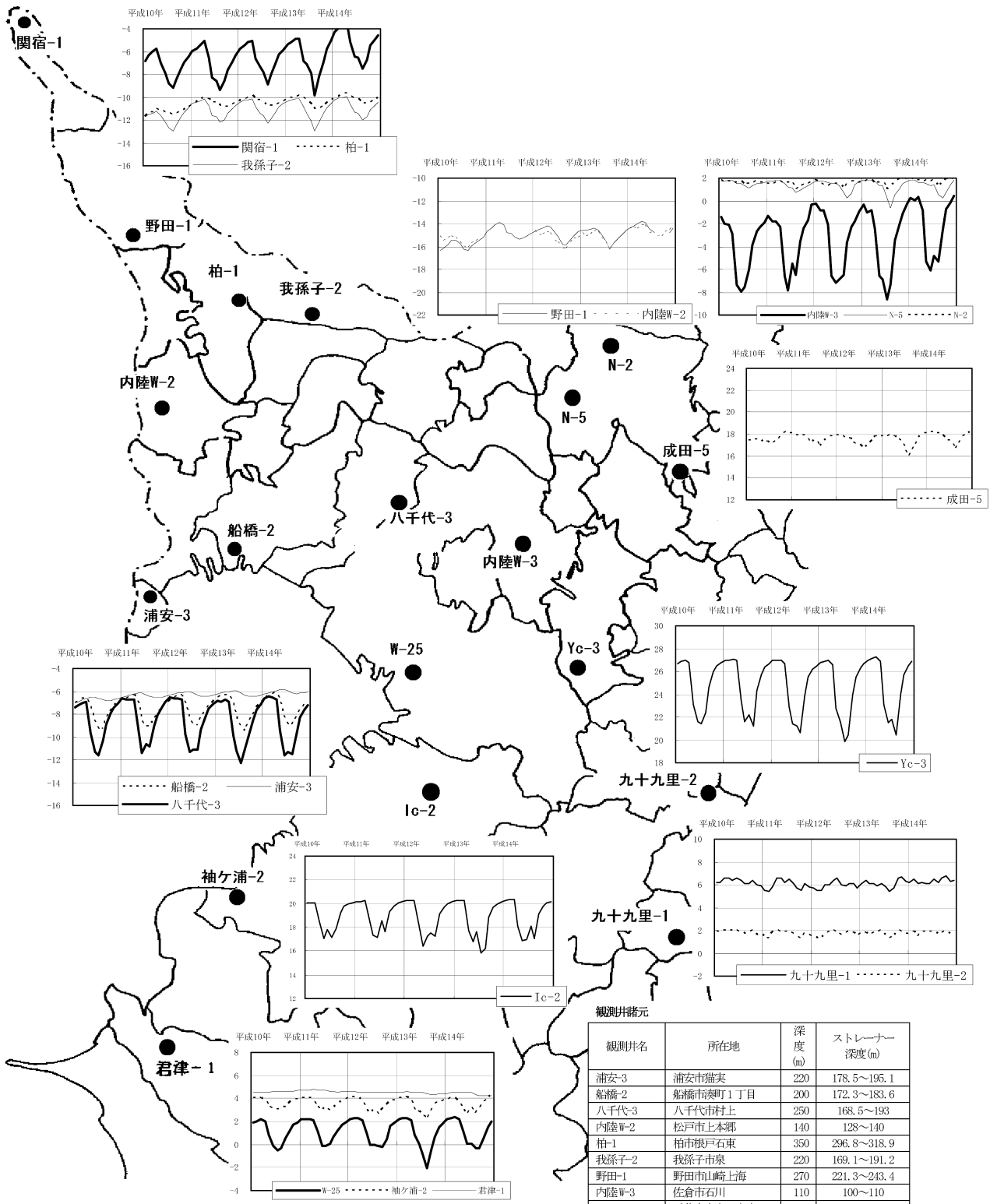
図2-10-5 地下水水位変動状況図
