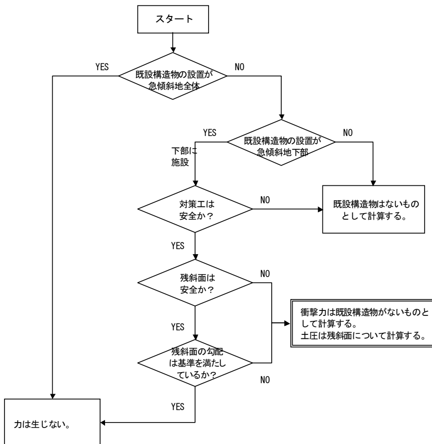
図 3.3 原因地対策が施工されている場合の評価フロー
