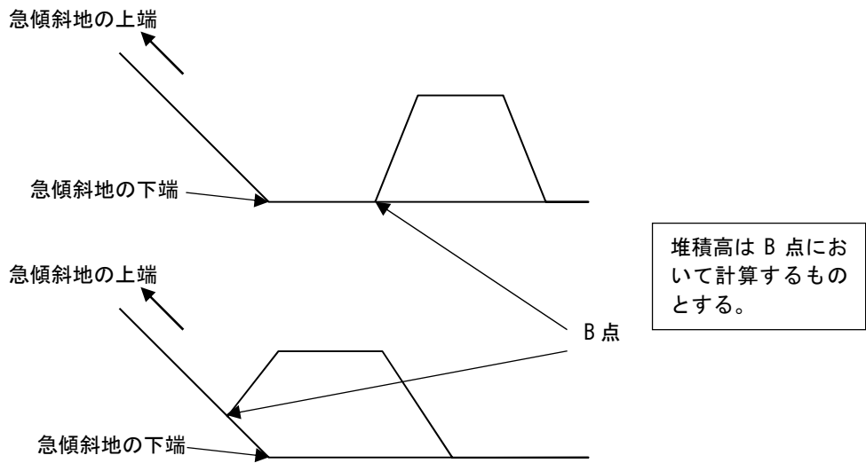
図 3.2 移動の力、堆積の力及び堆積高の計算位置
