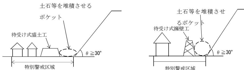
図 2.5 待受け式盛土工及び待受け式擁壁工のイメージ
