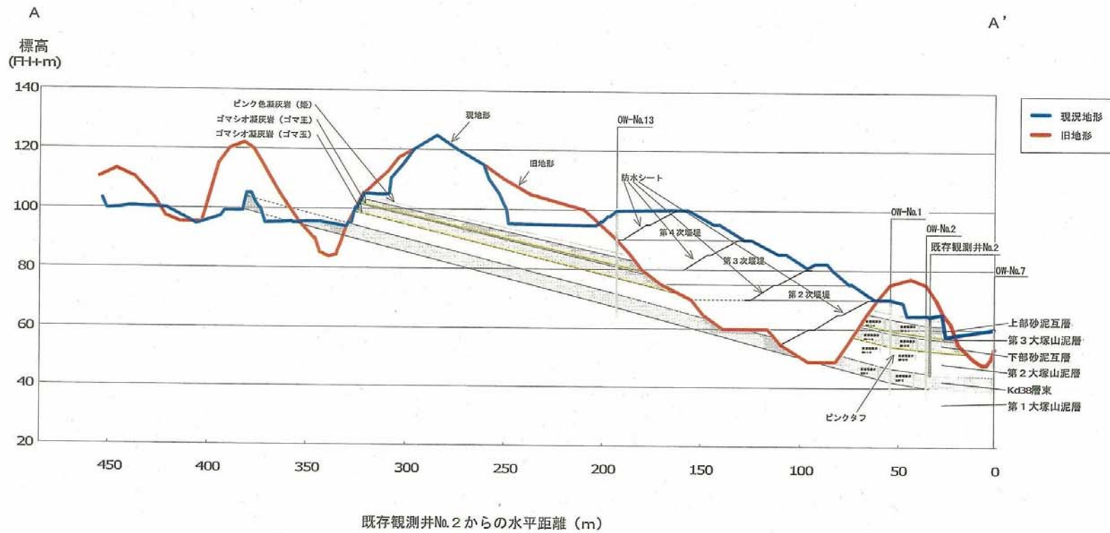
図-3 水文地質断面図
