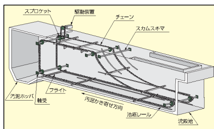
汚泥掻寄機
