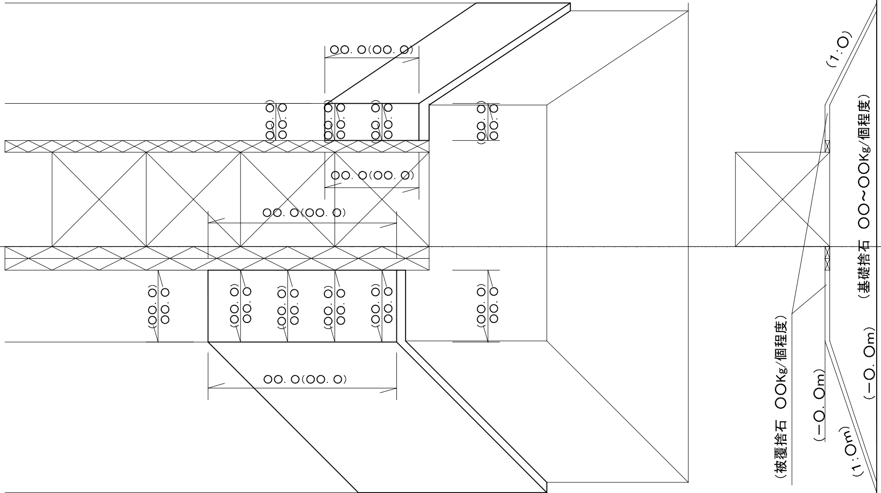
平面図
