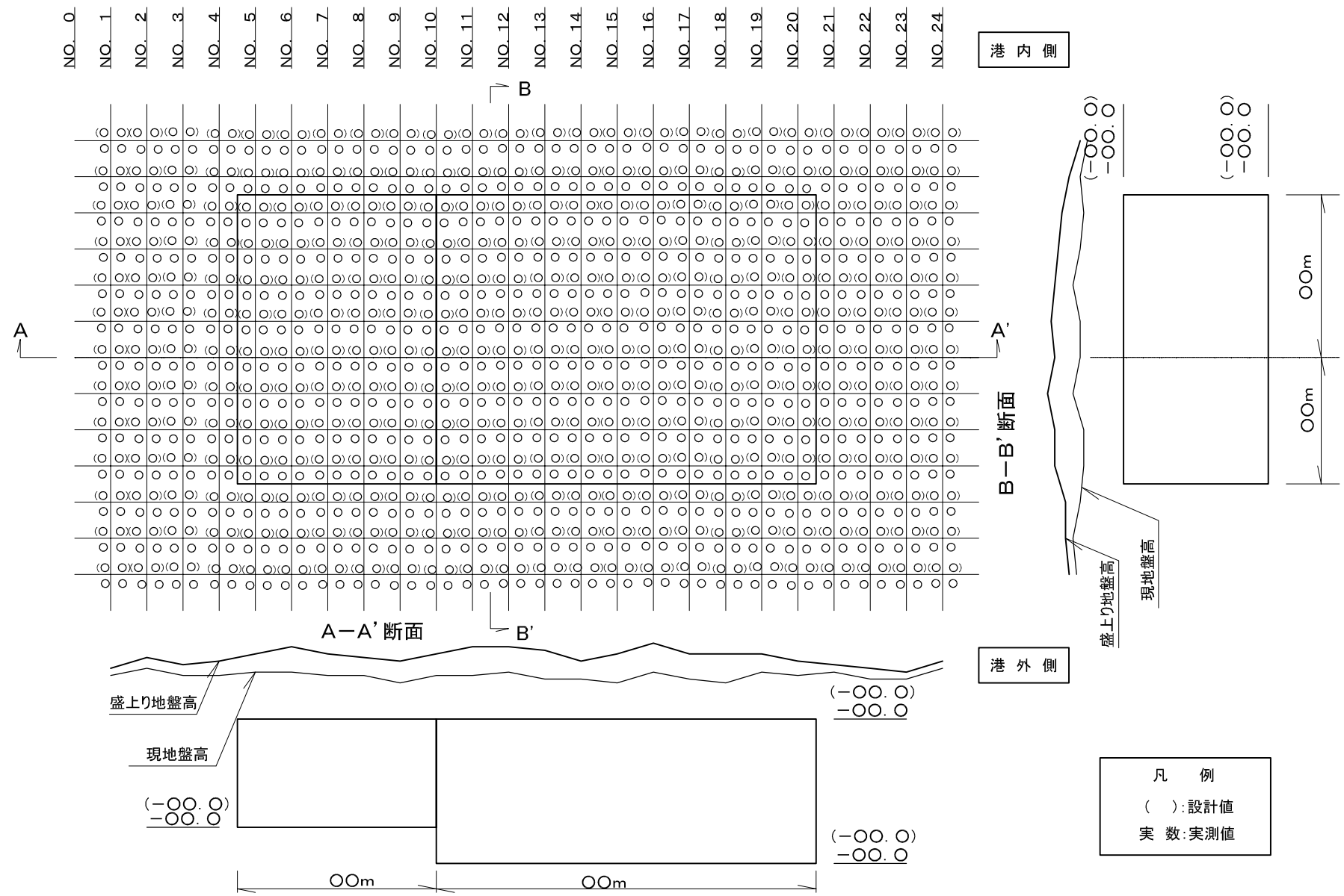
平面図
