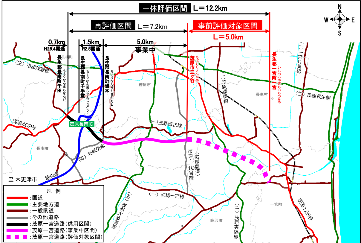
【計画平面図】
