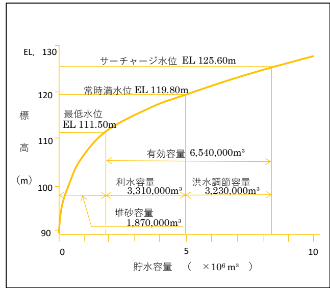
貯水位 - 容量曲線
