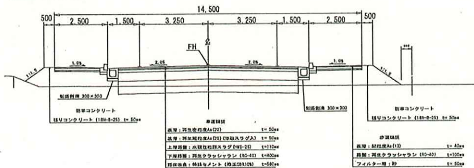
標準横断面図
