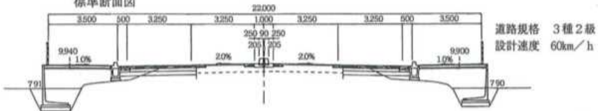
標準断面図
