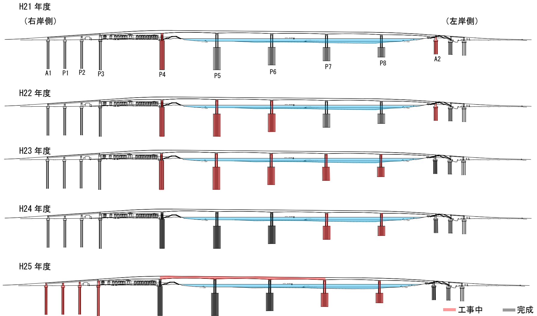
図 2-4 (1) 工事の施工実施順序
