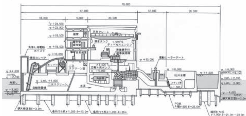
【海老川排水機場縦断面図】
