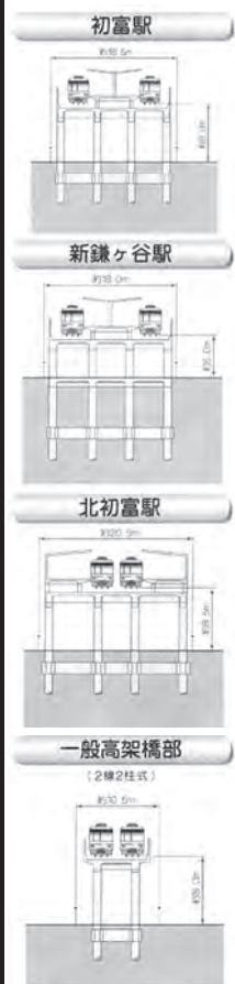
標準断面図
