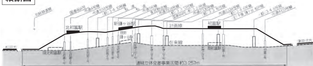
縦断面図
