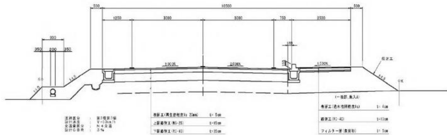
標準横断図 S=1:50
