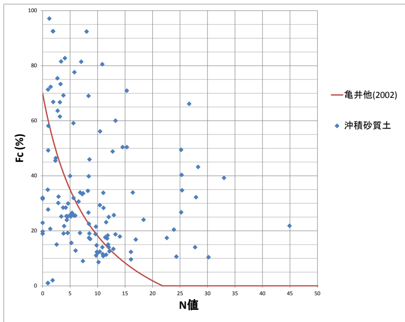
図-3.5.3 本調査 No.1~20 の沖積砂質土の N 値と細粒土含有率 Fc(%)との関係
