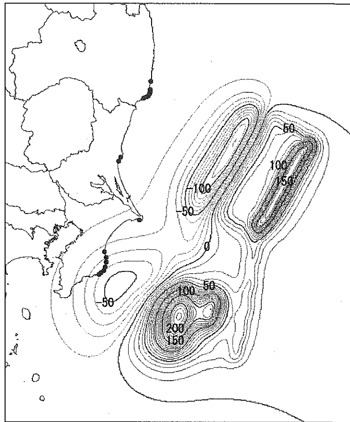
図2 延宝房総沖地震の断層モデルに基づく地盤変動量分布(単位:cm) (海岸の●印は図3に示した津波浸水高と計算遡上高の比較地点)
