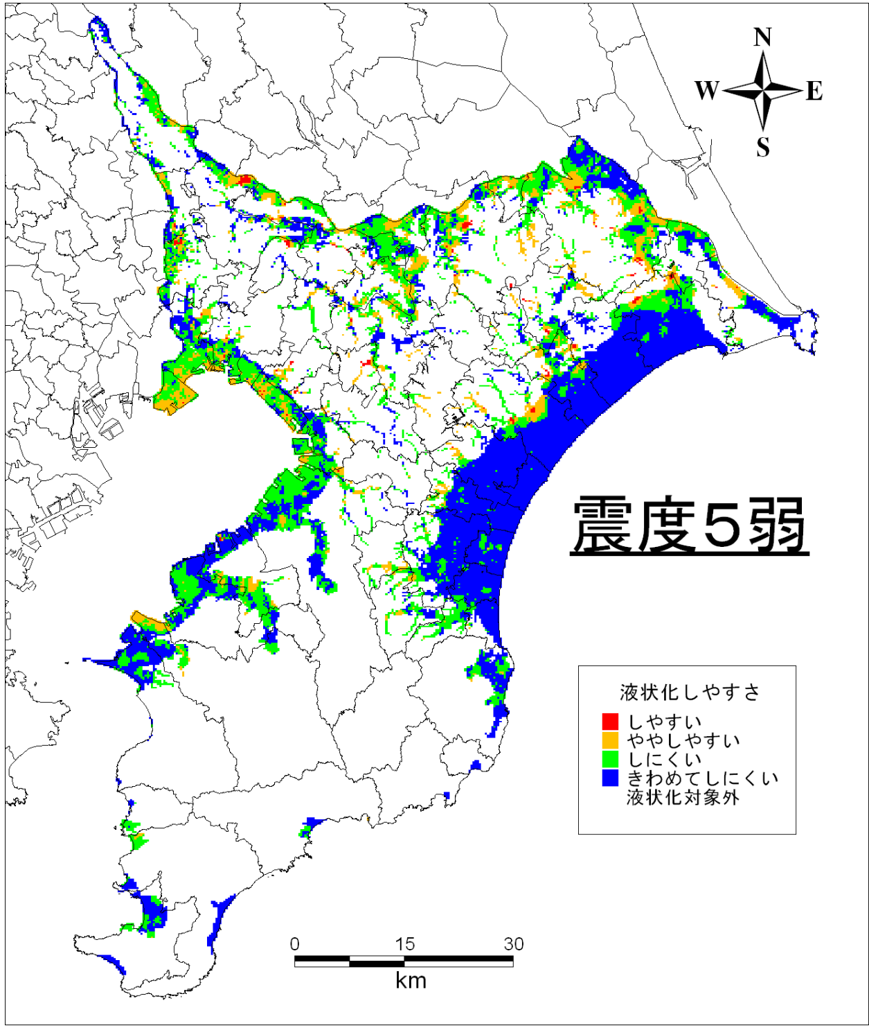
液状化しやすさ試算結果（震度5弱・地表加速度170gal・全県）
