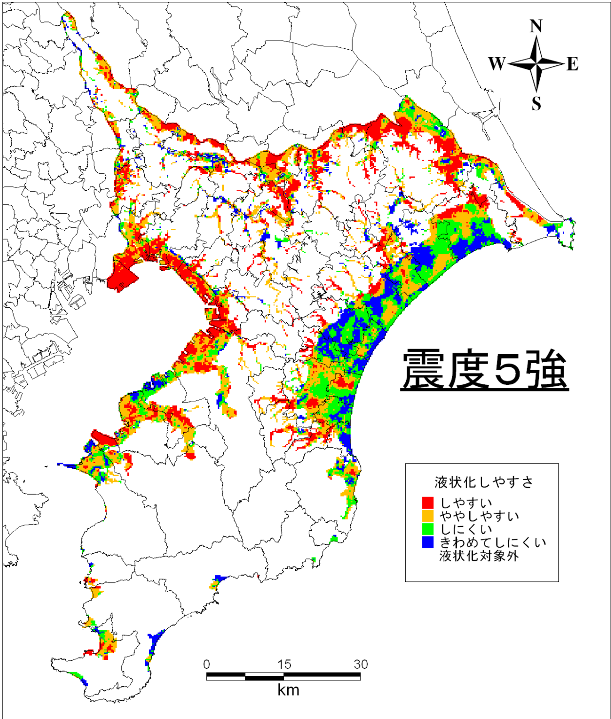
液状化しやすさ試算結果（震度5強・地表加速度340gal・全県）
